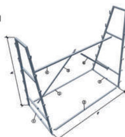
Стенд двосторонній для вхідних дверей Секції: 2 шт. Ширина: 26 см Висота: 245 см Глибина: 102 см Ширина дверей: 860/ 960 мм
