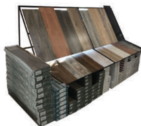
Стенд телескопічний для ламінату Секції: 16-32 планки Ширина: 166-310 см Висота: 150 см Глибина: 125 см
